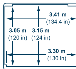
Main deck cargo door (STA 1770) Left-hand side
